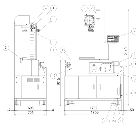
外形寸法図及び各部の名称
