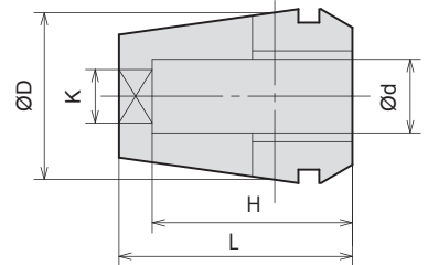
シャンクスルー仕様 Thru-the-shank coolant type
