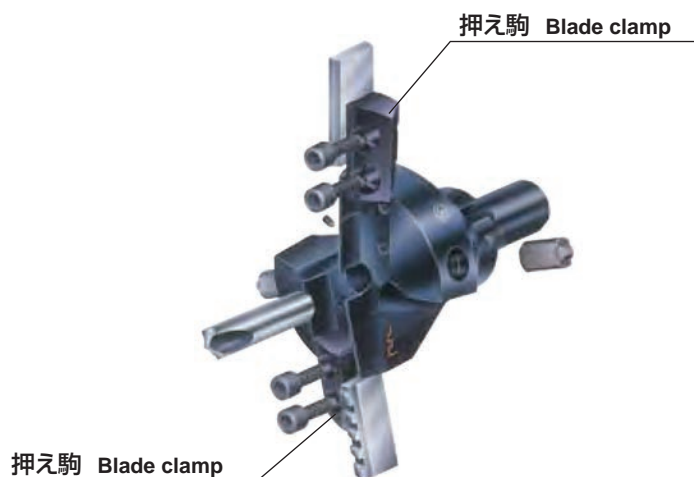
2個セット (ネジ付き) 2 pc set with screws
